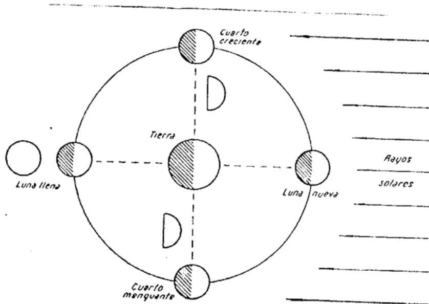
Fig. 10. Fases de la Luna
