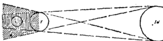
Fig. 12. Teoría del eclipse de Luna
