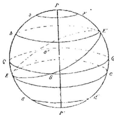
Fig. 4. Los elementos de la esfera celeste, PP', eje del mundo. QQ', ecuador celeste. aa', bE', Ec, dd', paralelos. Pa'E'Q'cd'P'dEQba, meridiano. EE', eclíptica. B, equinoccio de primavera. B', equinoccio de otoño. E, solsticio de invierno. E', solsticio de verano.
