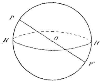
Fig. 3. HH', horizonte. P, polo norte celeste. P', polo sur celeste. PP', eje del mundo. PH'P'H, esfera celeste
